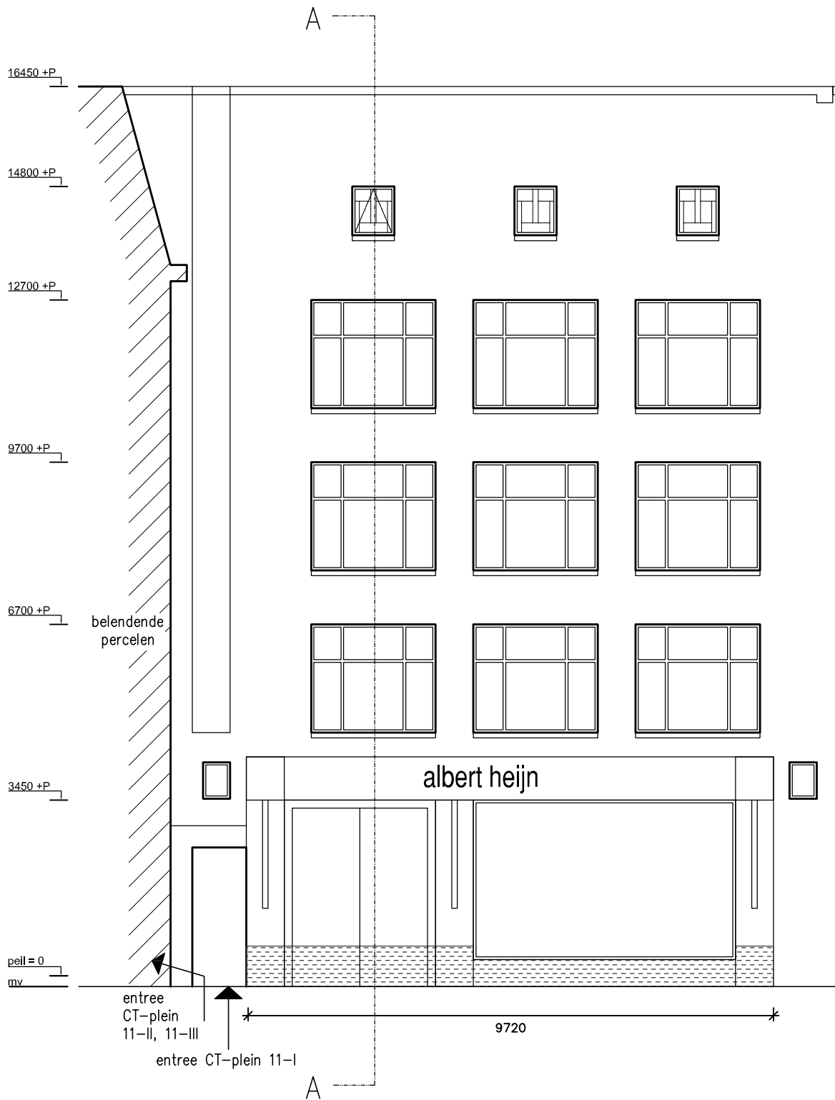
vooraanzicht best. = nw. situatie
