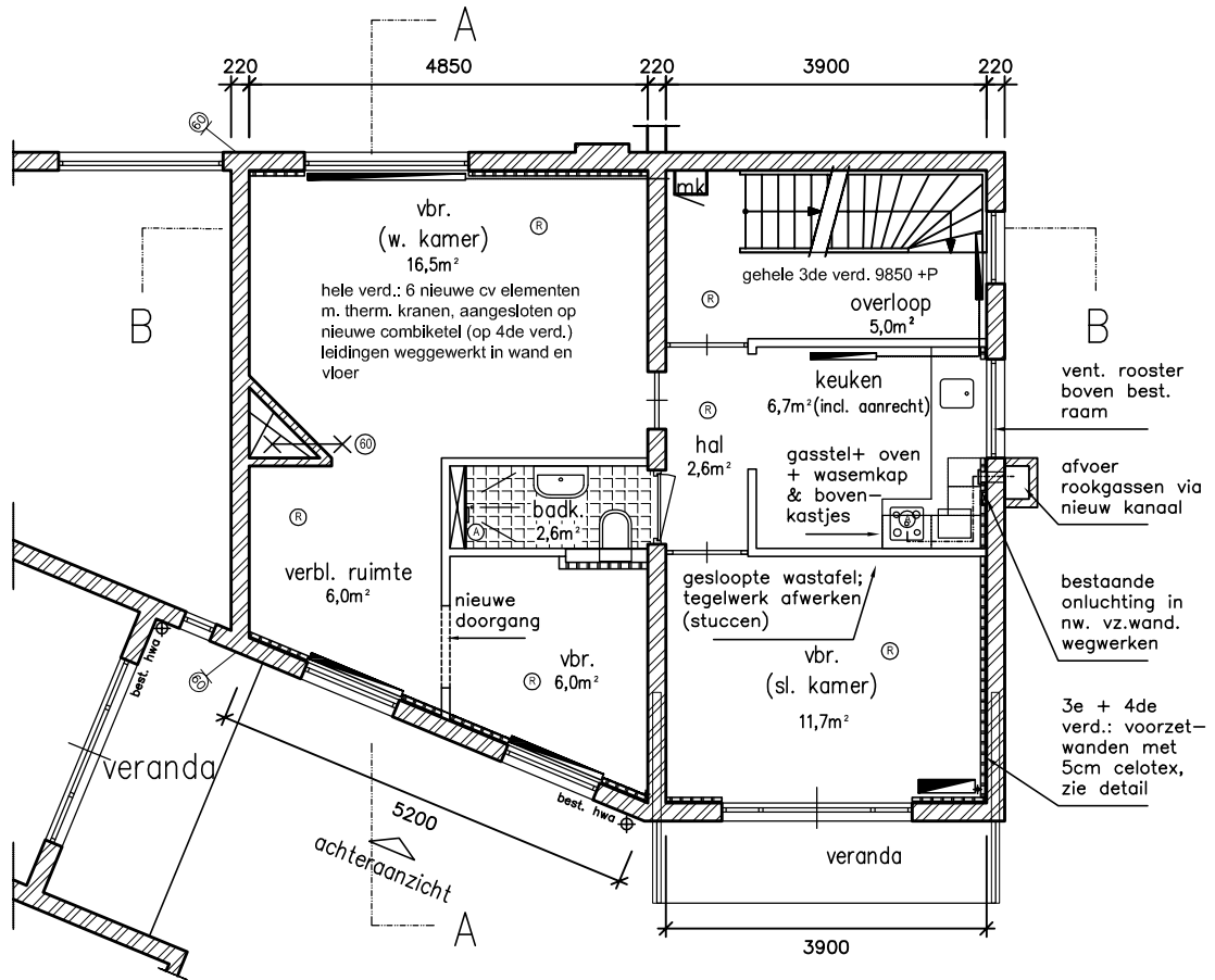
3de verdieping nieuwe situatie
