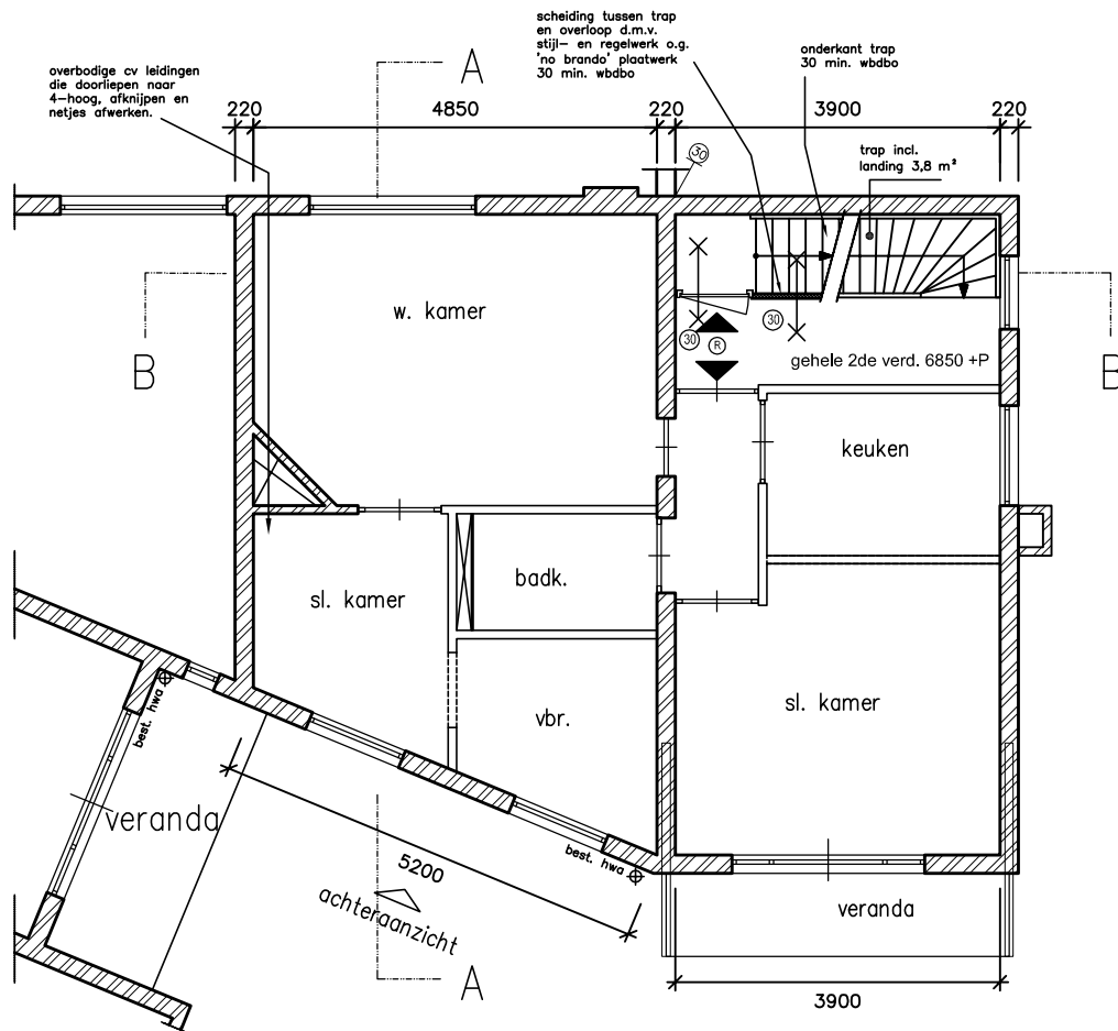
2de verdieping nieuwe situatie
